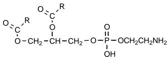
2-aminoethyl phosphatidates
